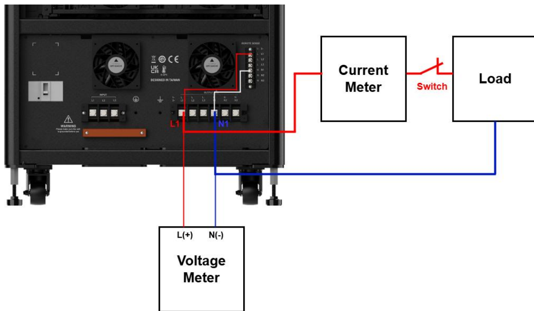
圖 8-1 校準設備接線(L1/N1)示意圖
