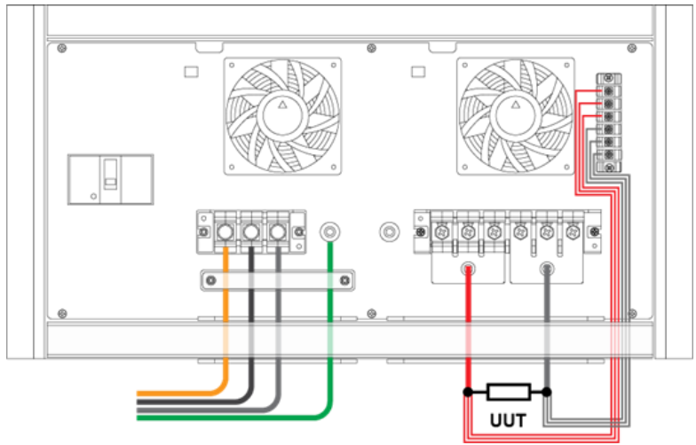
圖 3-7 單相模式輸出和遠端量測線接線方式
