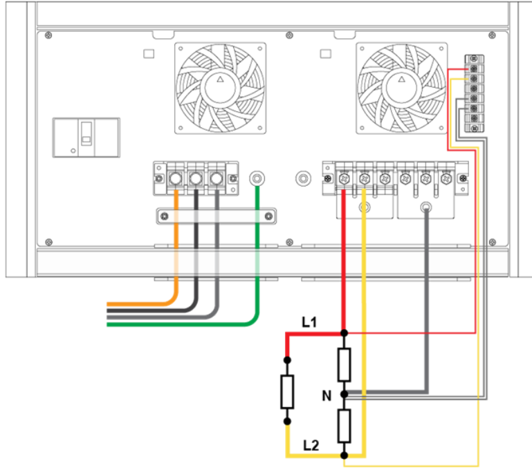
圖 3-8 分相模式輸出和遠端量測線接線方式
