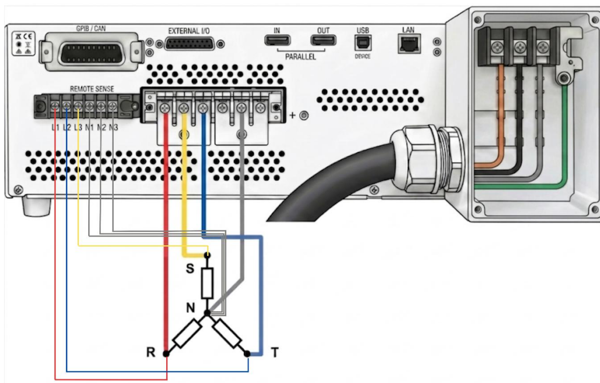
圖 3-6 三相模式輸出和遠端量測線接線方式
