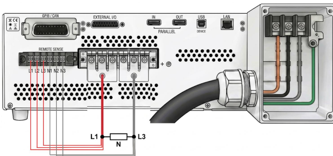
圖 3-7 單相模式輸出和遠端量測線接線方式
