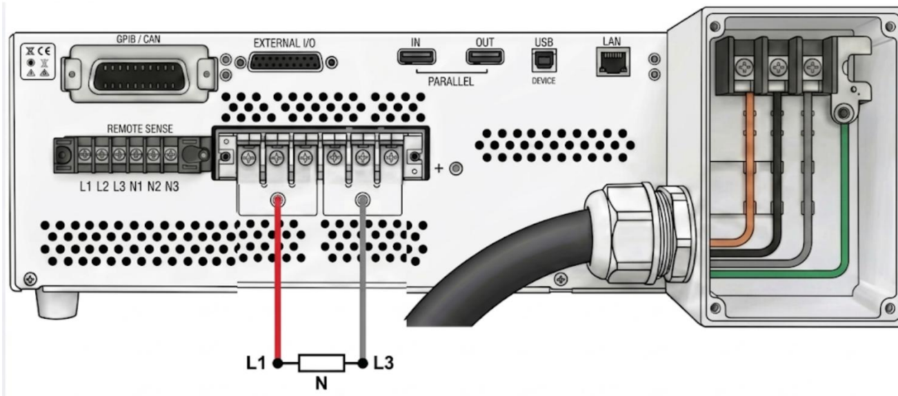
圖 3-4 輸出單相模式接線方式
