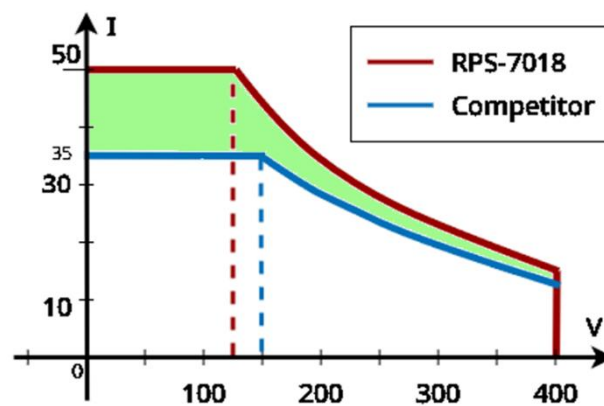
圖 1-1 交流電壓/電流操作範圍圖-三相模式
