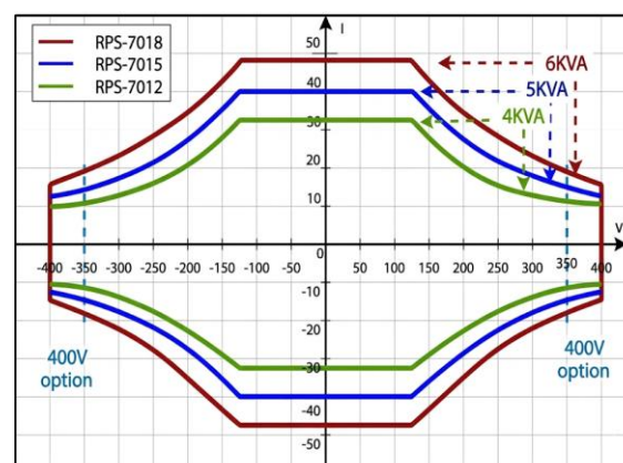
圖 1-2 直流電壓/電流操作範圍圖-單相模式
