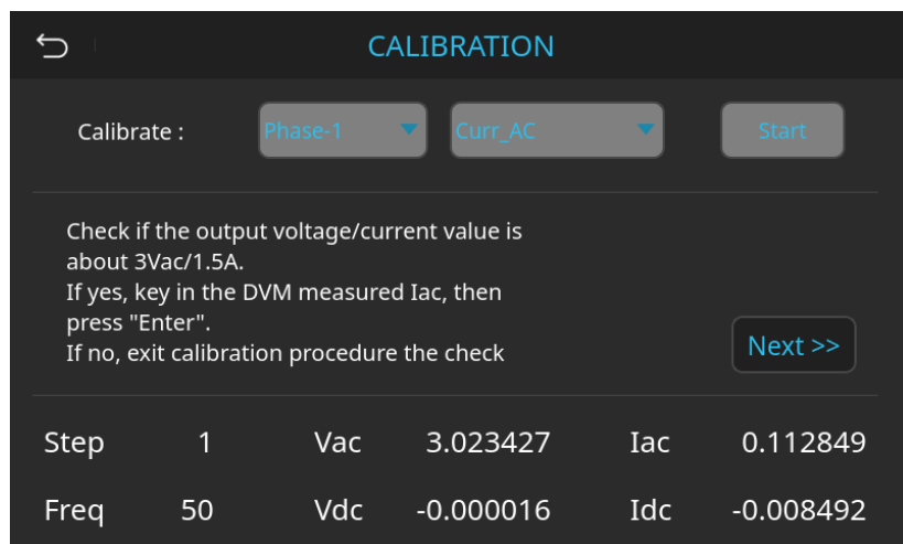
圖 8-22 校準輸出交流電流程式-輸出 3Vac
