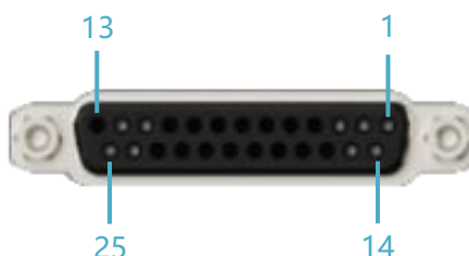
圖 11-1 External I/O 端子編號示意圖
