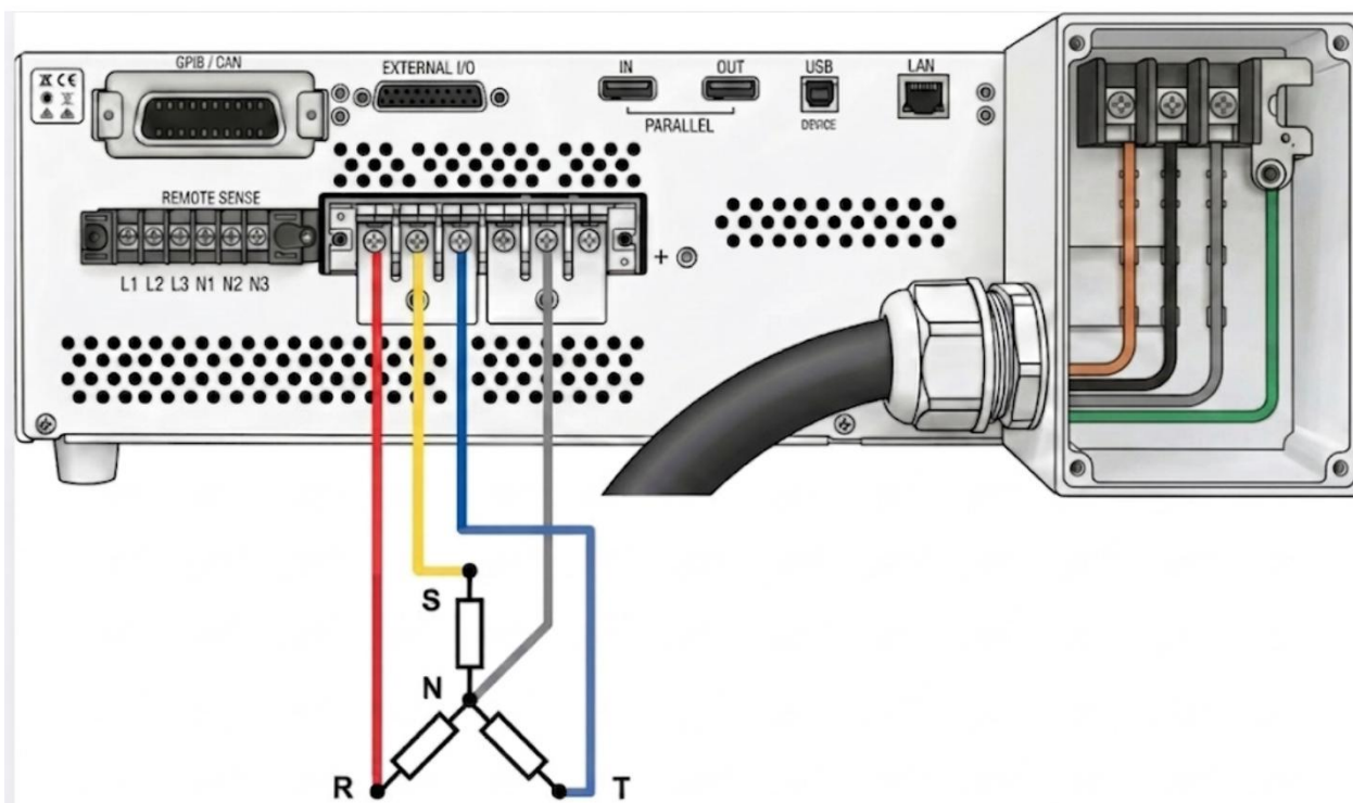
圖 3-3 輸出三相模式接線方式
