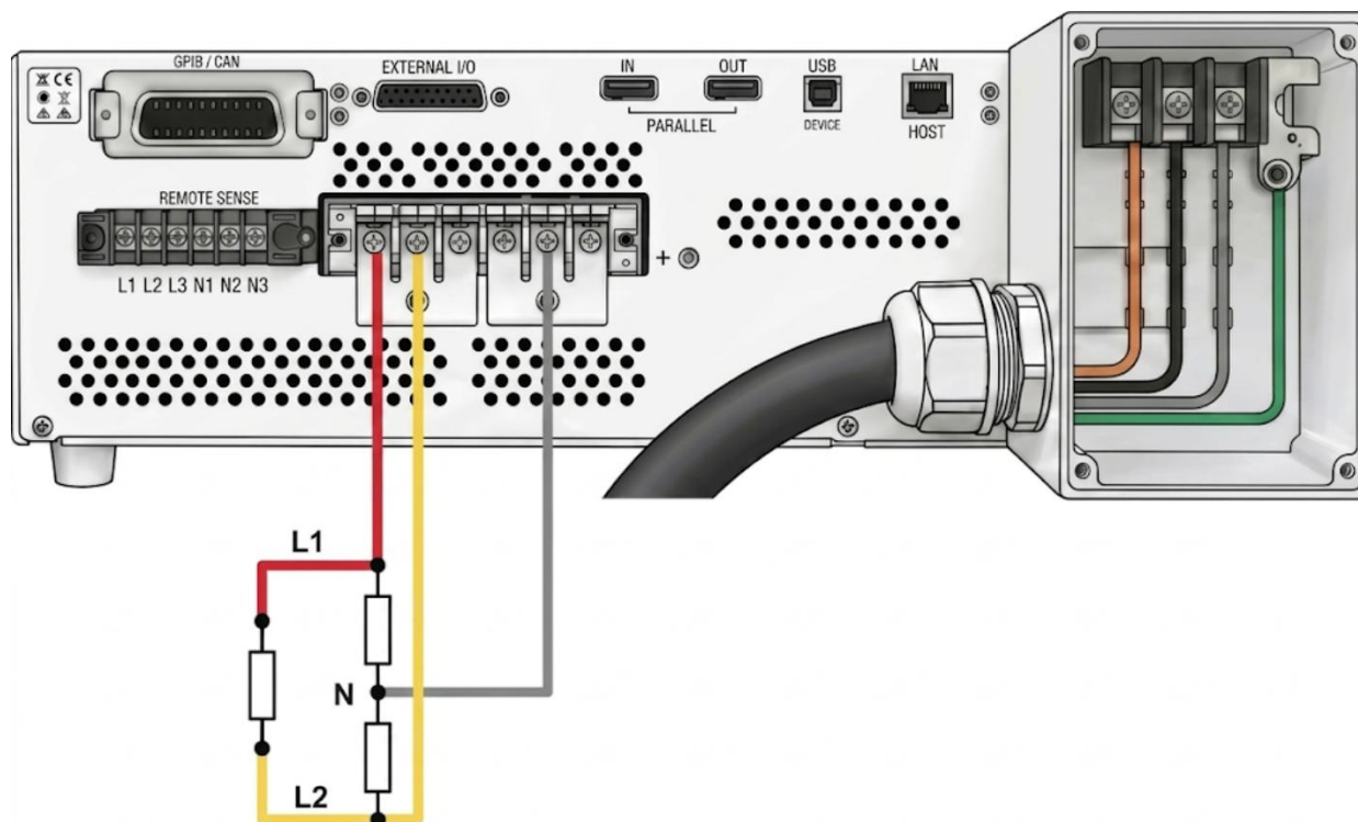
圖 3-5 輸出分相模式接線方式
