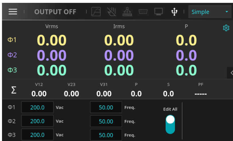
圖 4-36 三相模式主畫面(Coupling=AC)
