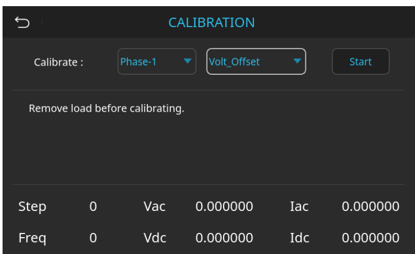
圖 8-5 校準第一相的輸出偏移電壓畫面
