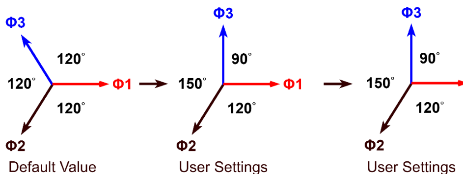
圖 4-33 輸出配置(Phase)頁面- Independent Relock 禁用時
