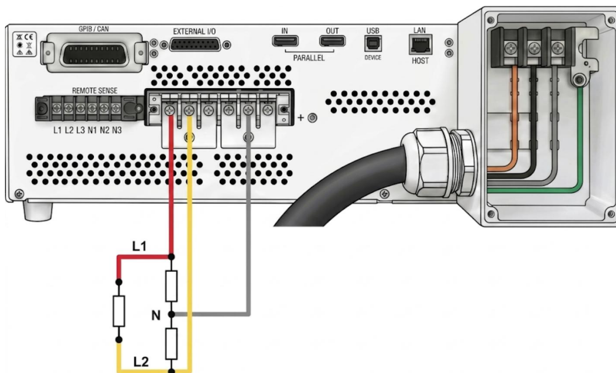
圖 3-5 輸出分相模式接線方式
