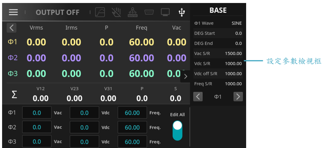
圖 4-14 三相 Base 模式下設定參數檢視框資訊
