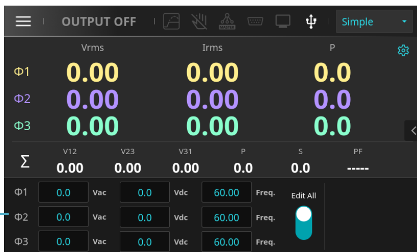
圖 4-5 三相模式基本參數設定欄位
