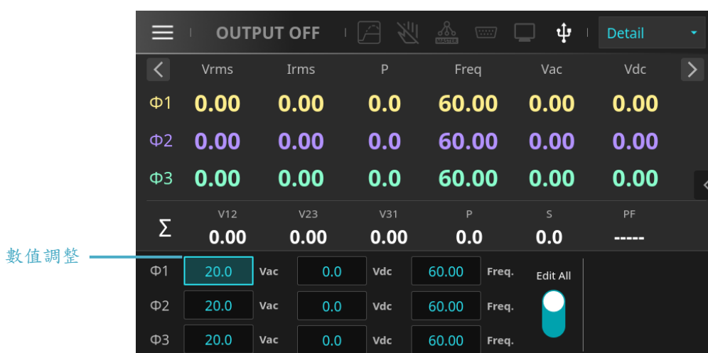
圖 4-8 按壓旋鈕進行數值調整
