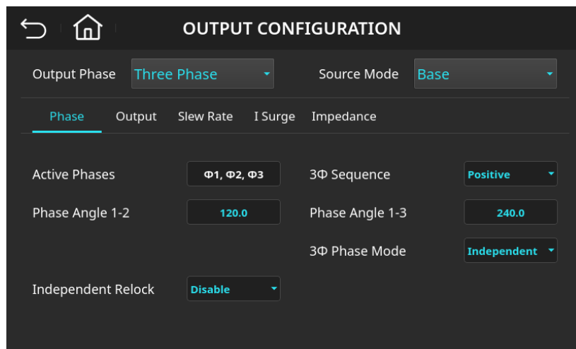
圖 4-21 輸出配置設定頁面
