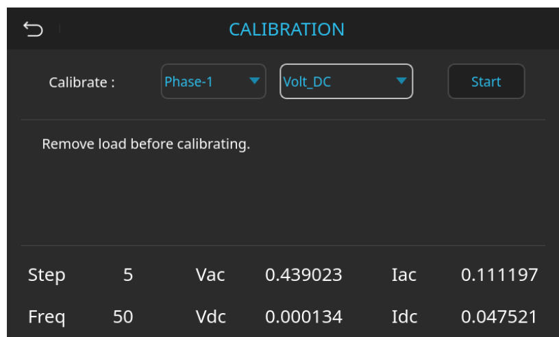
圖 8-11 校準第一相的輸出直流電壓畫面
