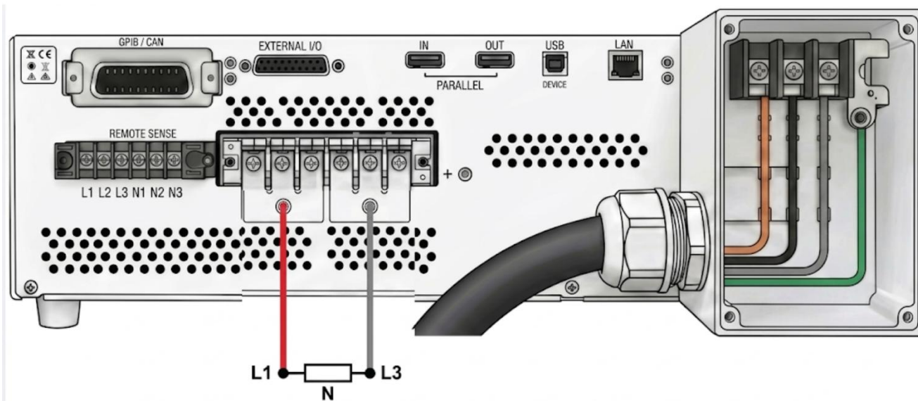
圖 3-4 輸出單相模式接線方式
