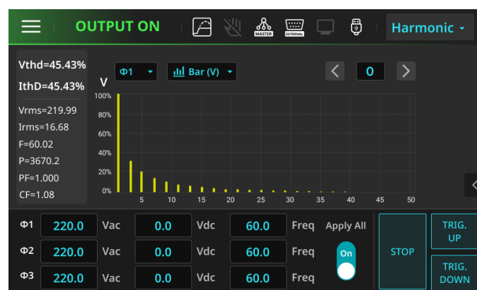
圖 9：高級諧波分析
