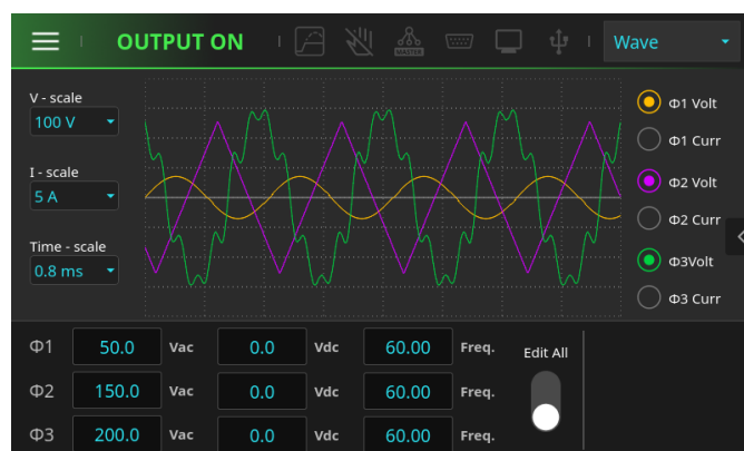
圖 8：三相電壓波形
