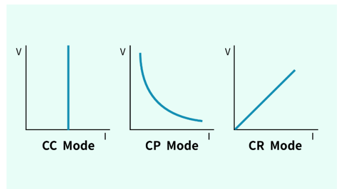
圖 2：多模式電子負載解決方案
